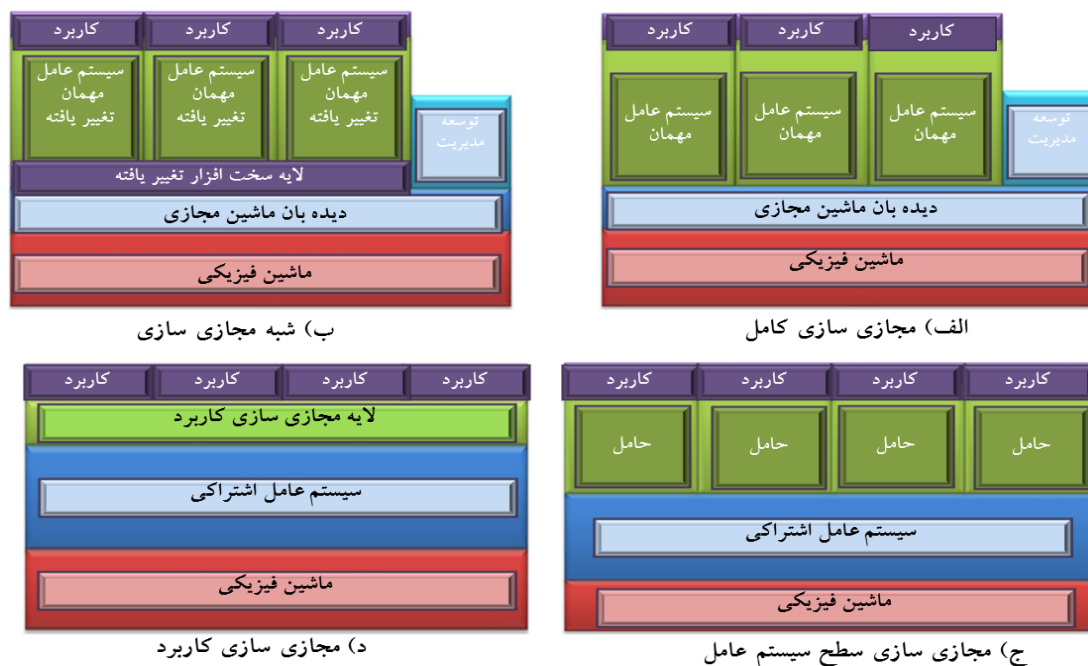
شکل ۳: تکنولوژی های مختلف مجازی سازی
